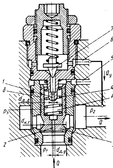
Рис. 1. Клапан непрямого действия
