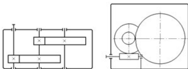
Кинематические схемы редукторов
