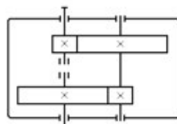
Кинематические схемы редукторов
