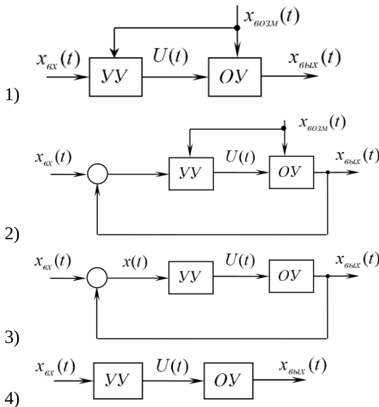
Структура САУ
