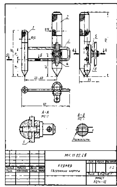
Рис. 72. Вариант 2: кернер служит для набивки углублений при разметке деталей. Он состоит из неподвижного 1 и подвижного 2 бойков, укреплённых на направляющей 3. Неподвижный боек соединён с направляющей благодаря расплыванию ее концов, а подвижный — с помощью планки 4 и винта 5, имею
