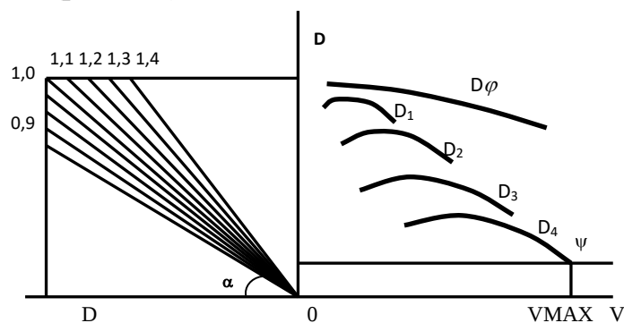
Рисунок 2.3 Универсальная динамическая характеристика
