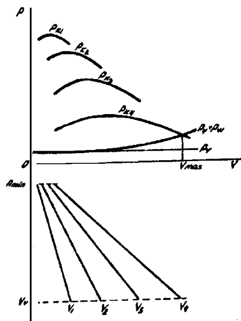
Рисунок 2.2 Тягово-скоростная характеристика автомобиля
